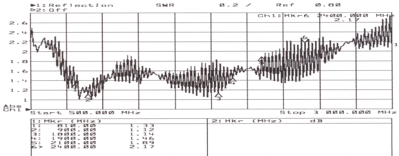
Figure 1 VSWR 500MHz - 3000MHz
